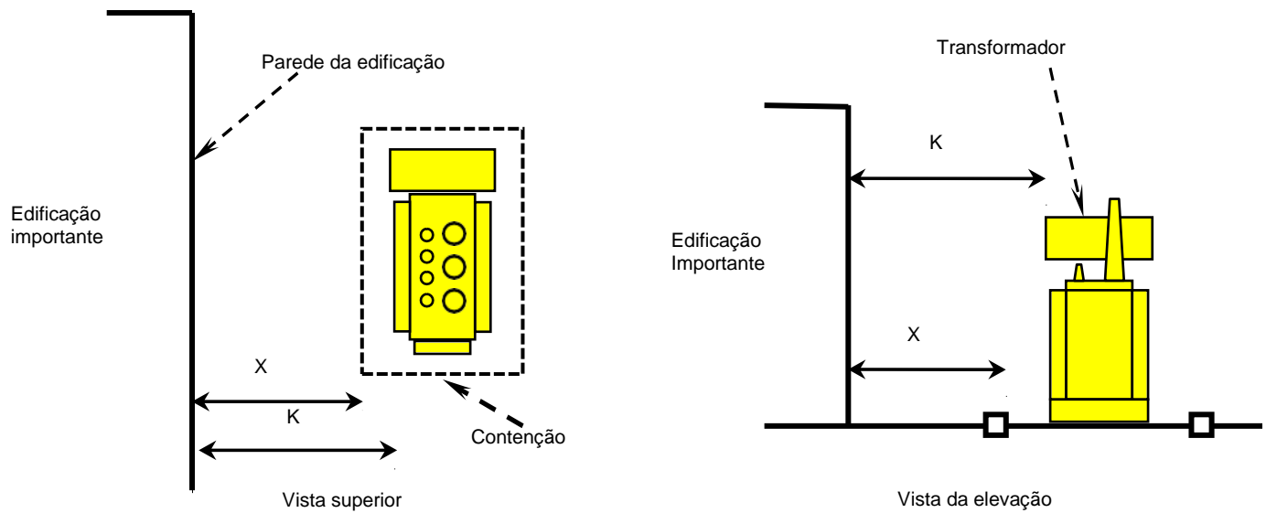
Figura A.4: Transformador imerso em líquido isolante instalado externamente a edificação
