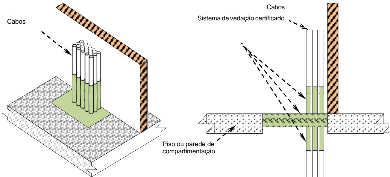
Figura A.1: Exemplo de vedação de abertura para passagem de cabos entre ambientes compartimentados
