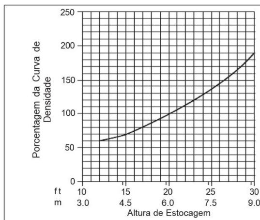
Figura 5.2.2.1.5.3: Densidade do sistema no teto vs. altura de armazenagem.
