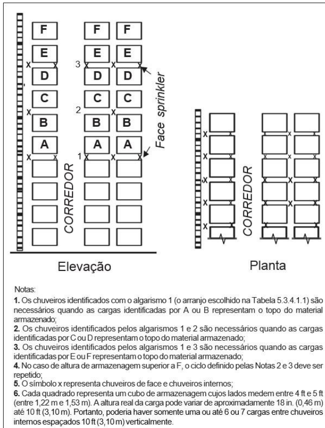
Figura 5.3.4.4.1(i): Distribuição de chuveiros internos, mercadorias Classe I, Classe II, Classe III ou Classe IV, altura de armazenagem acima de 7,6 m (25 ft) – Opção 2.
