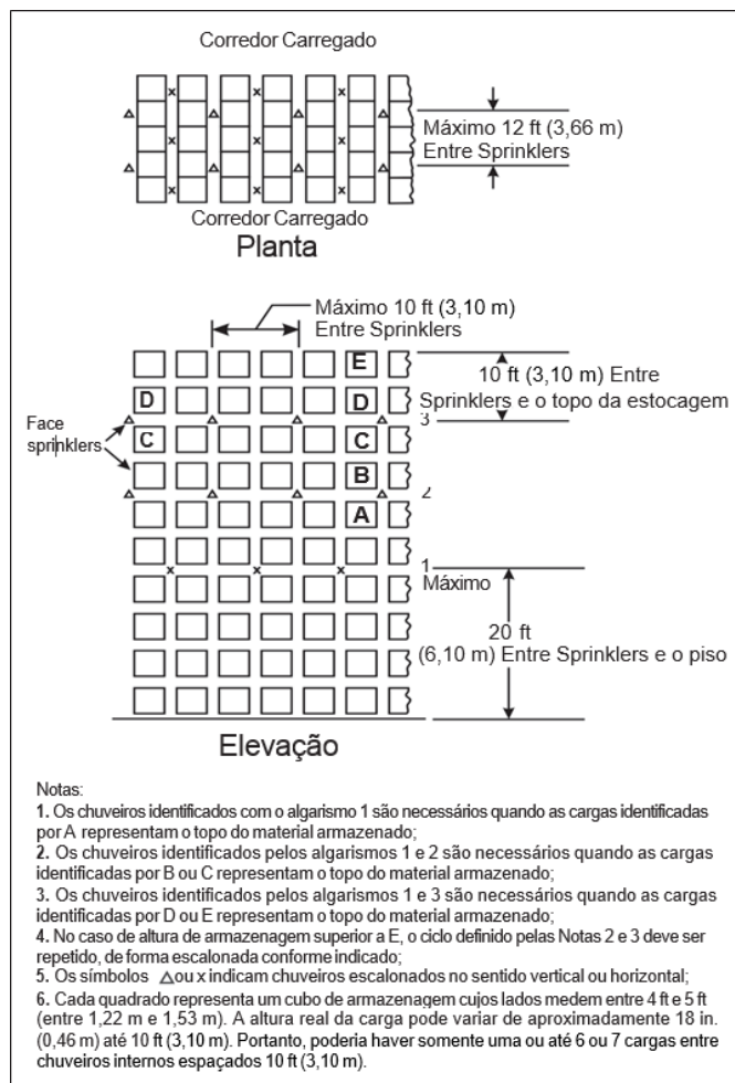
Figura 5.3.4.4.1.3(a): Distribuição de chuveiros internos, estruturas porta-paletes múltiplas, mercadorias Classe I, altura de armazenagem acima de 7,6 m (25 ft)
