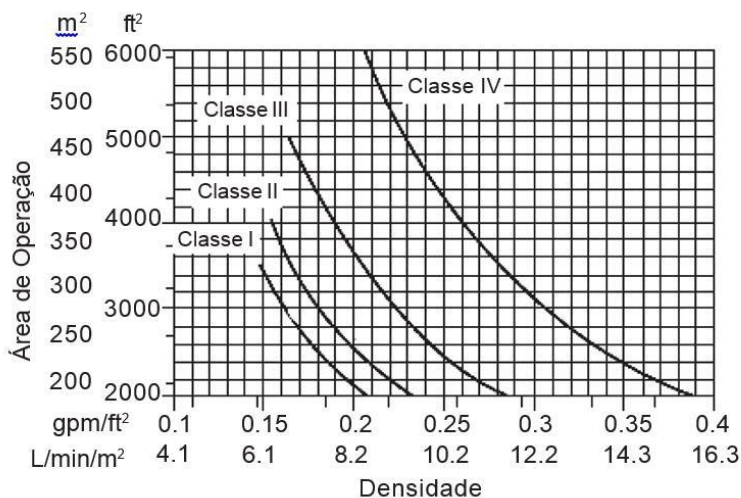
Figura 5.2.2.1.5.1: Curvas de projetos de sistemas de chuveiros, armazenagem 6,1 m (20 ft) de altura – chuveiros de temperatura normal.
