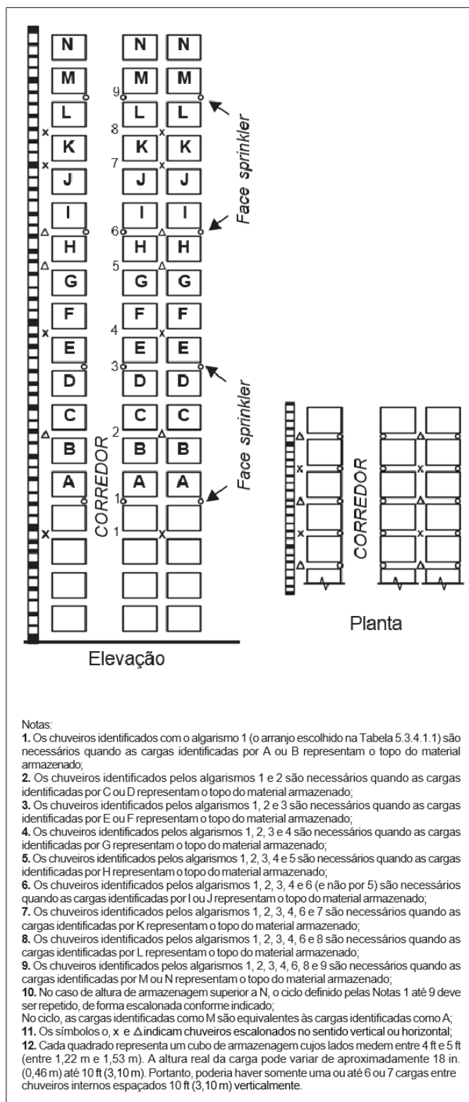
Figura 5.3.4.4.1(h): Distribuição de chuveiros internos, mercadorias Classe I, Classe II, Classe III ou Classe IV, altura de armazenagem acima de 7,6 m (25 ft) – Opção 1.
