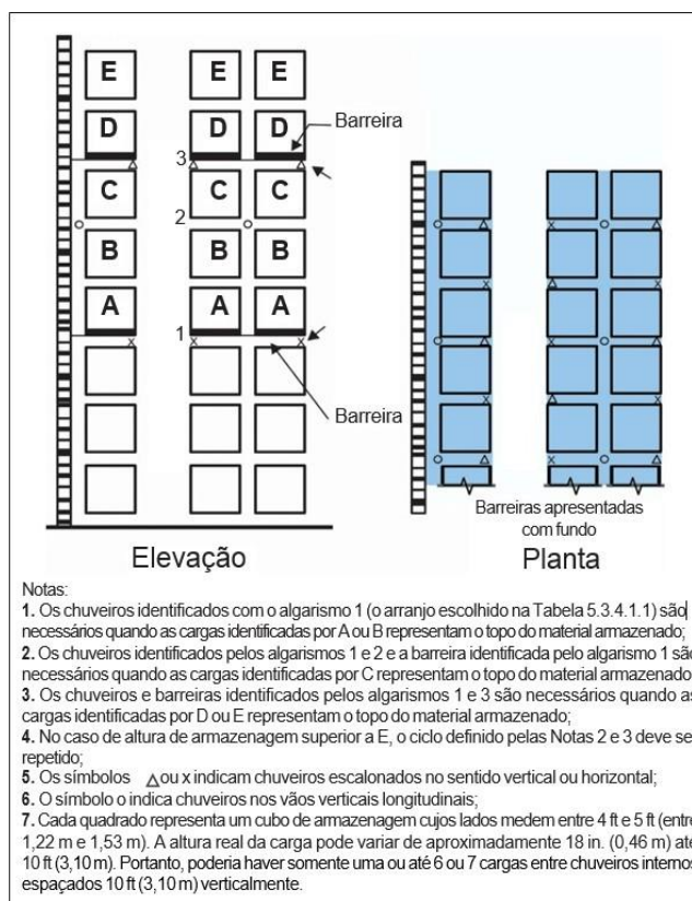
Figura 5.3.4.4.1(j): Distribuição de chuveiros internos, mercadorias Classe I, Classe II, Classe III ou Classe IV, altura de armazenagem acima de 7,6 m (25 ft) – Opção 3.
