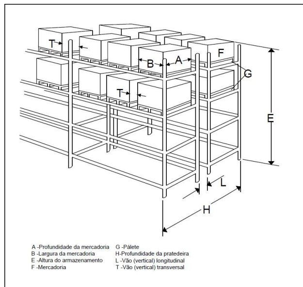
Figura E.8: Estruturas porta-paletes
