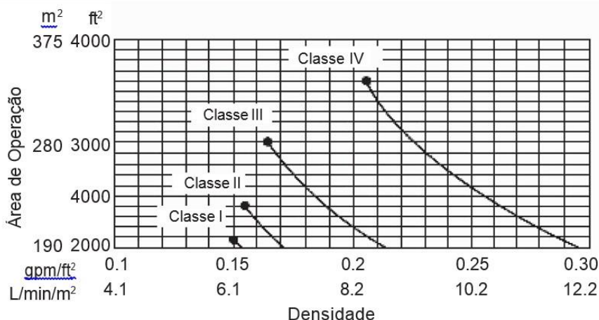
Figura 5.2.2.1.5.2: Curvas de projetos de sistemas de chuveiros, armazenagem a 6,1 m (20 ft) de altura – chuveiros de temperatura alta.
