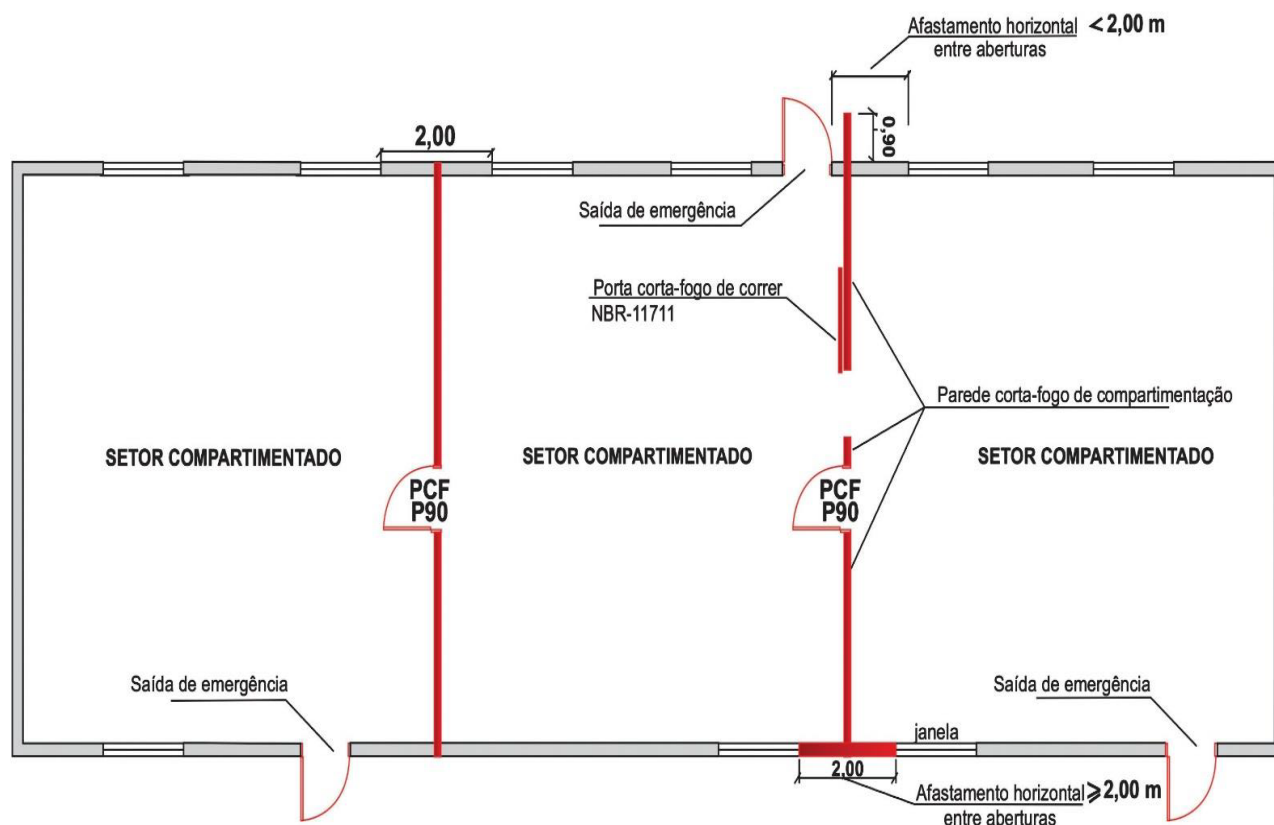
Figura A1: Modelo de compartimentação horizontal.
