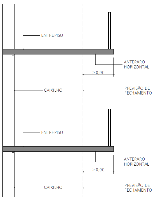
Figura A7: Modelo de fechamento com vidro.
