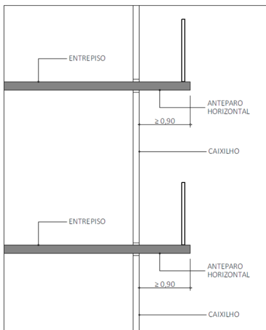
Figura A3: Modelo de compartimentação vertical.
