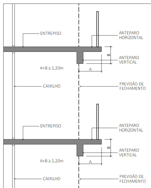
Figura A9: Modelo de fechamento com vidro.
