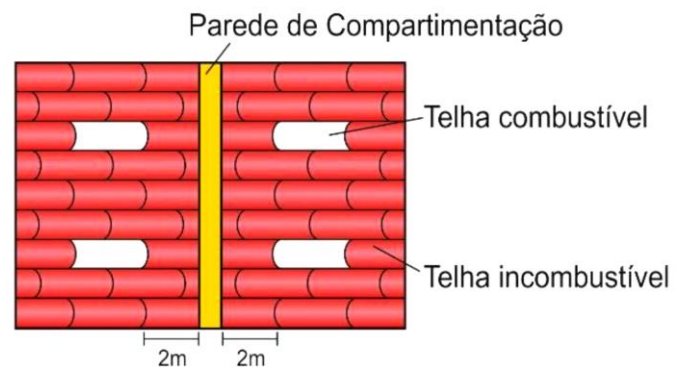
Figura 1: Afastamento de telhas combustíveis.
