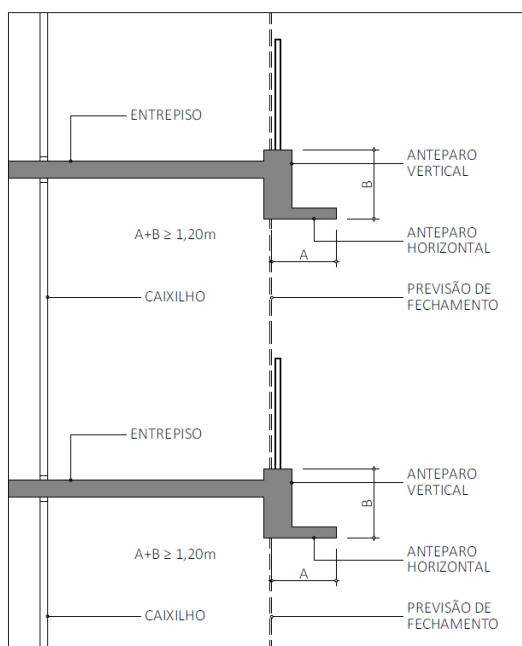
Figura A8: Modelo de fechamento com vidro.
