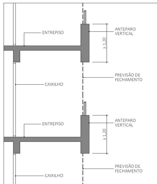
Figura A6: Modelo de fechamento com vidro.
